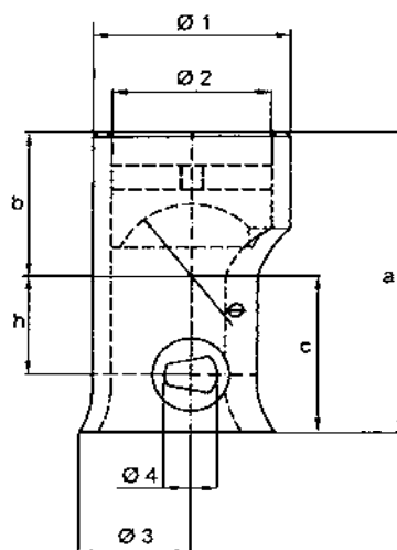
element suport sfera "3000" -Tip 2.
