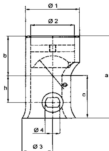
Serie cuzinet sfera "3000" -Tip 1.
