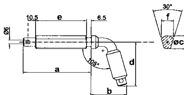
Bolt siguranta Tip1.
