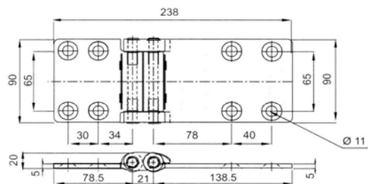
5101-095-4
