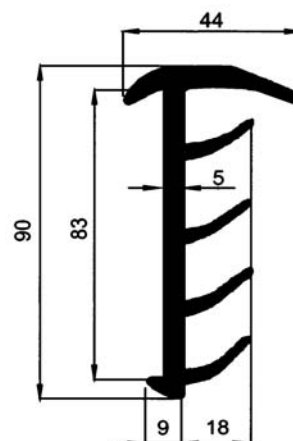
5109-82-16
