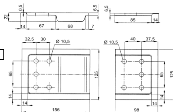
5101-115-4
