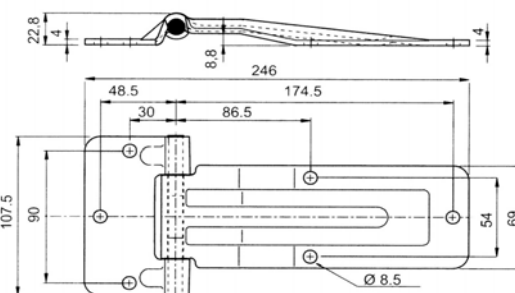
5101-111-4
