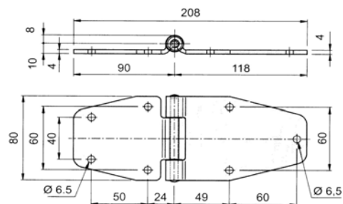
5101-080-4
