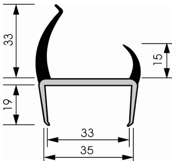
5108-35-17
