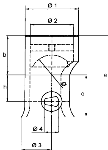
Guľové sedlo série "3000" - 2. typ
